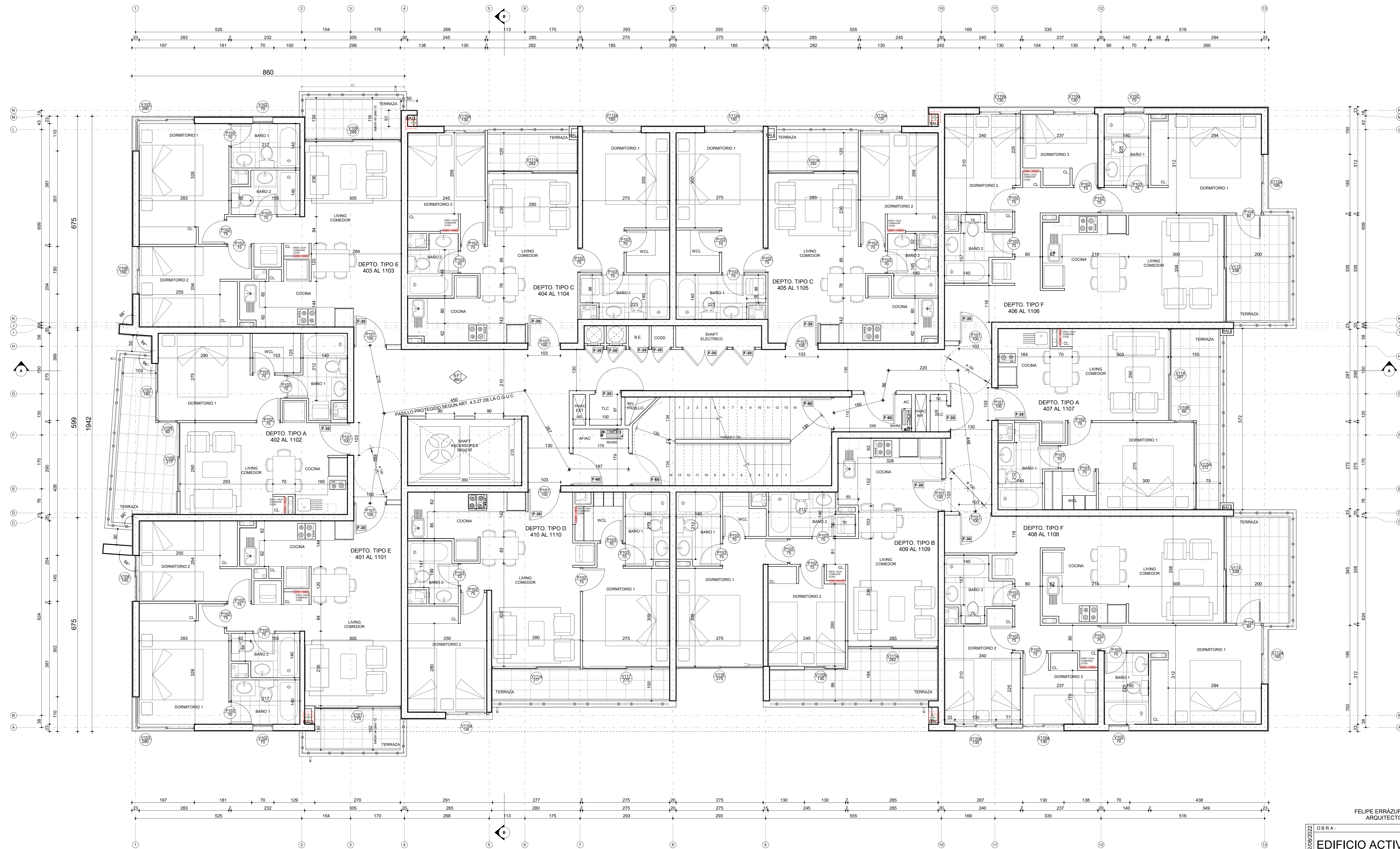
PLANTA TIPO DEL 4º AL 12º PISO ESCALA 1 : 50
