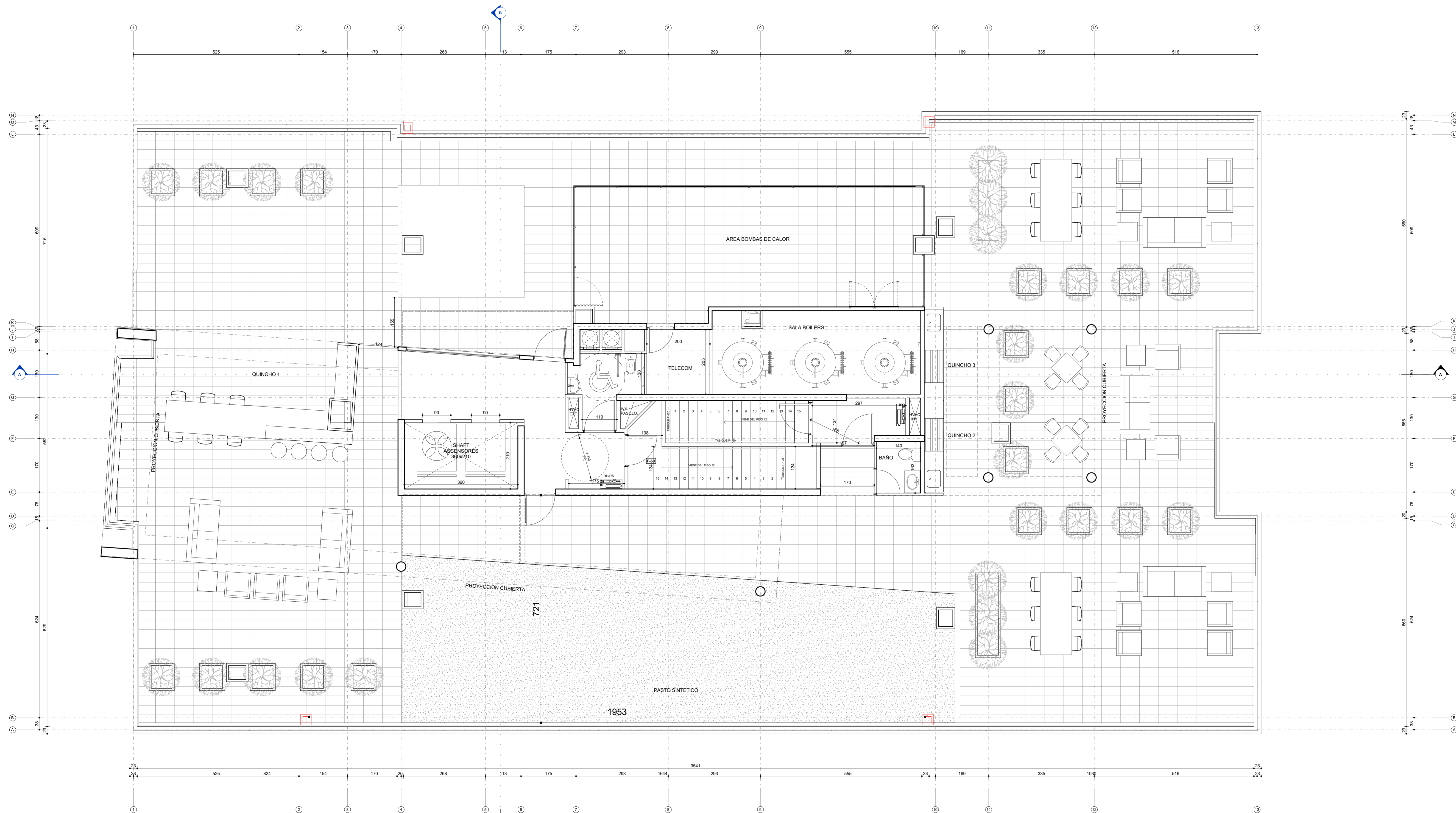
PLANTA PISO MIRADOR ESCALA 1:50
