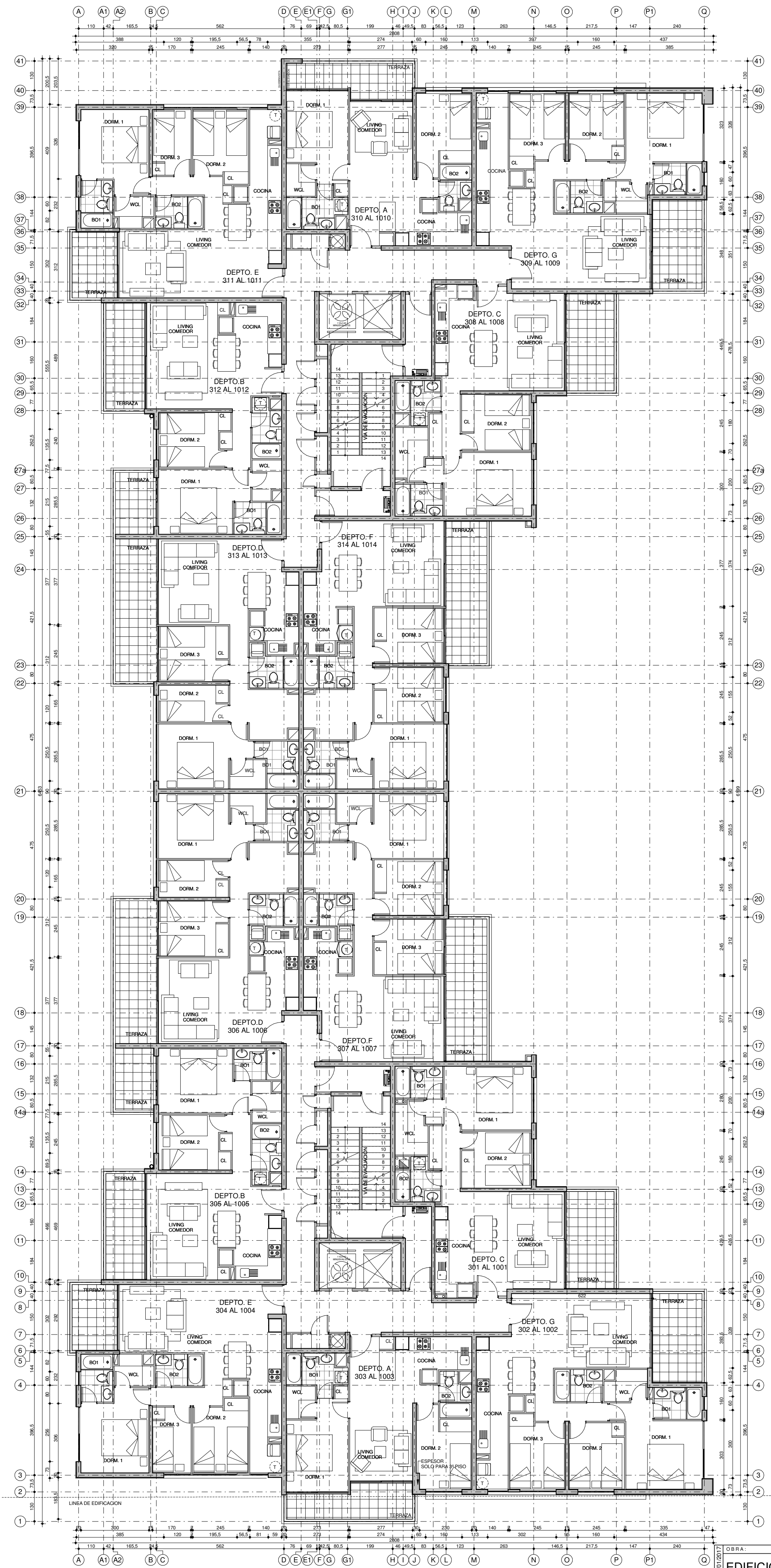
PLANTA TIPO DEL 3º AL 10º PISO
