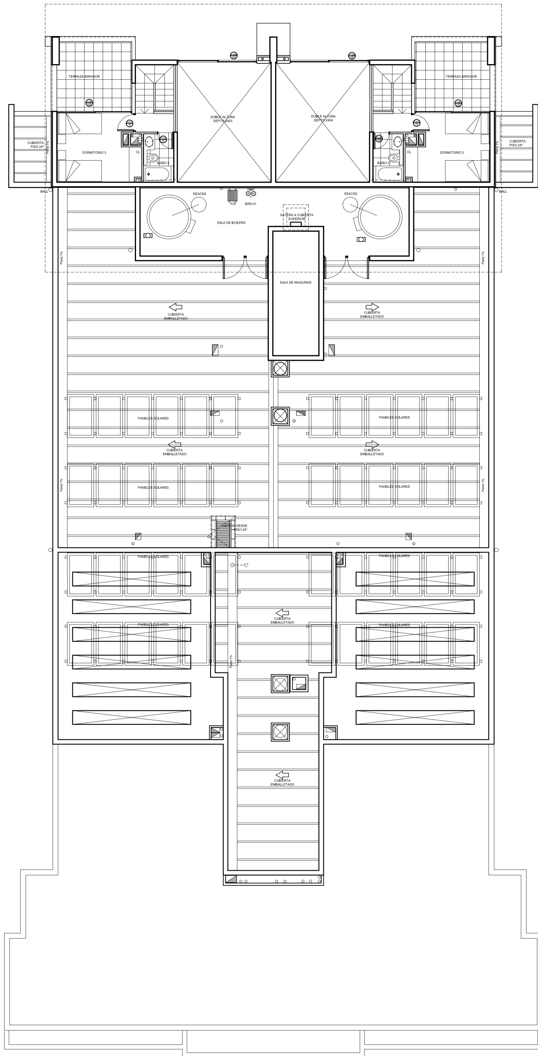
PLANTA DE ARQUITECTURA PISO MIRADOR
