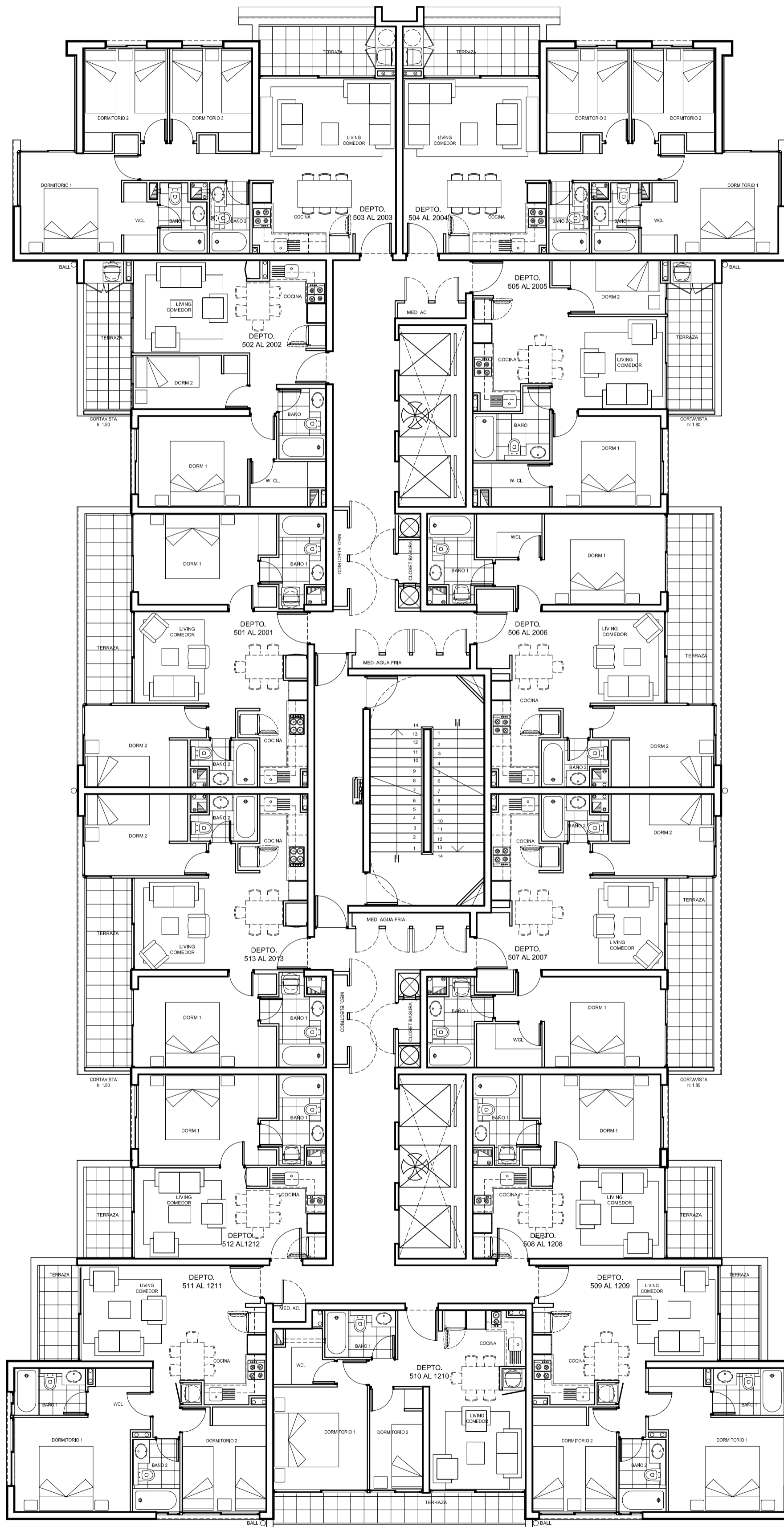
PLANTA DE ARQUITECTURA 5° AL 12° PISO
