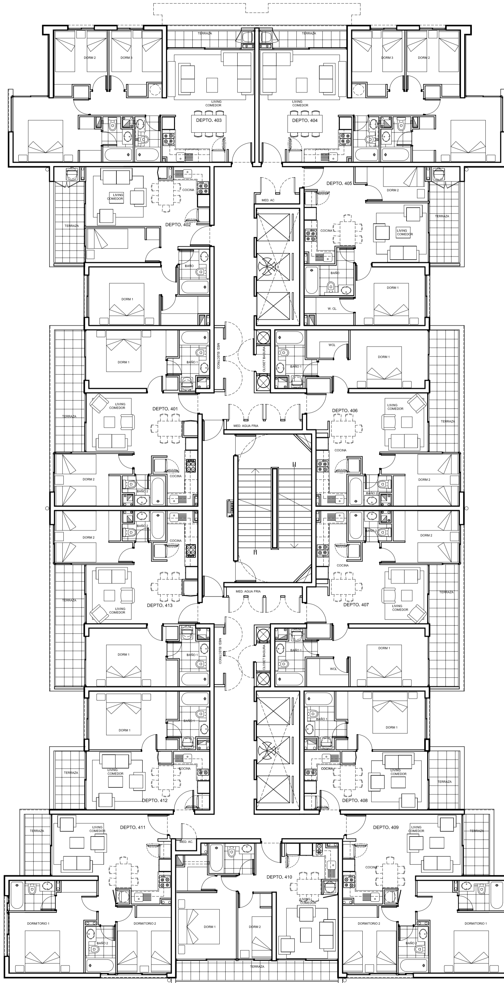
PLANTA DE ARQUITECTURA 4ºPISO
