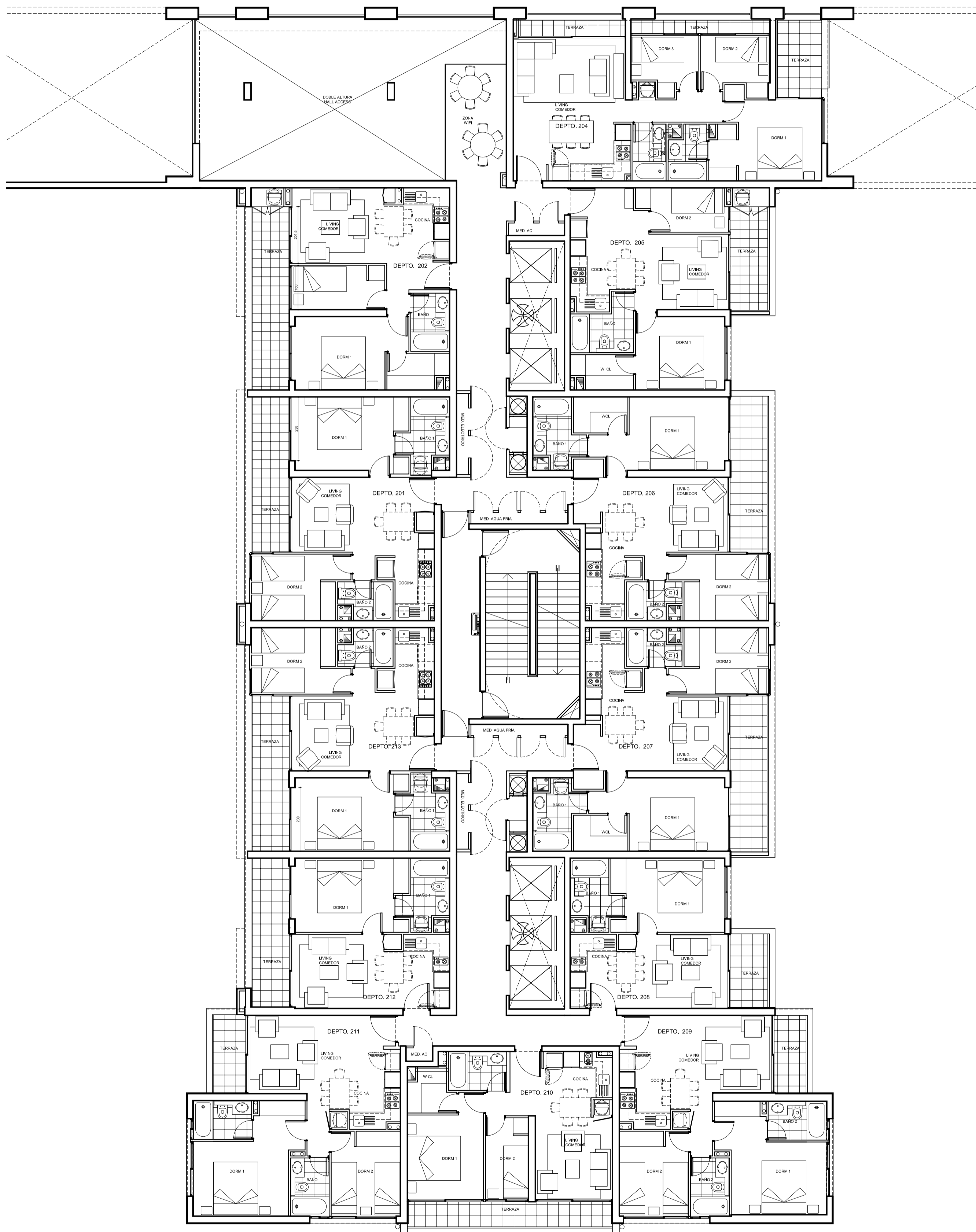
PLANTA DE ARQUITECTURA 2° PISO
