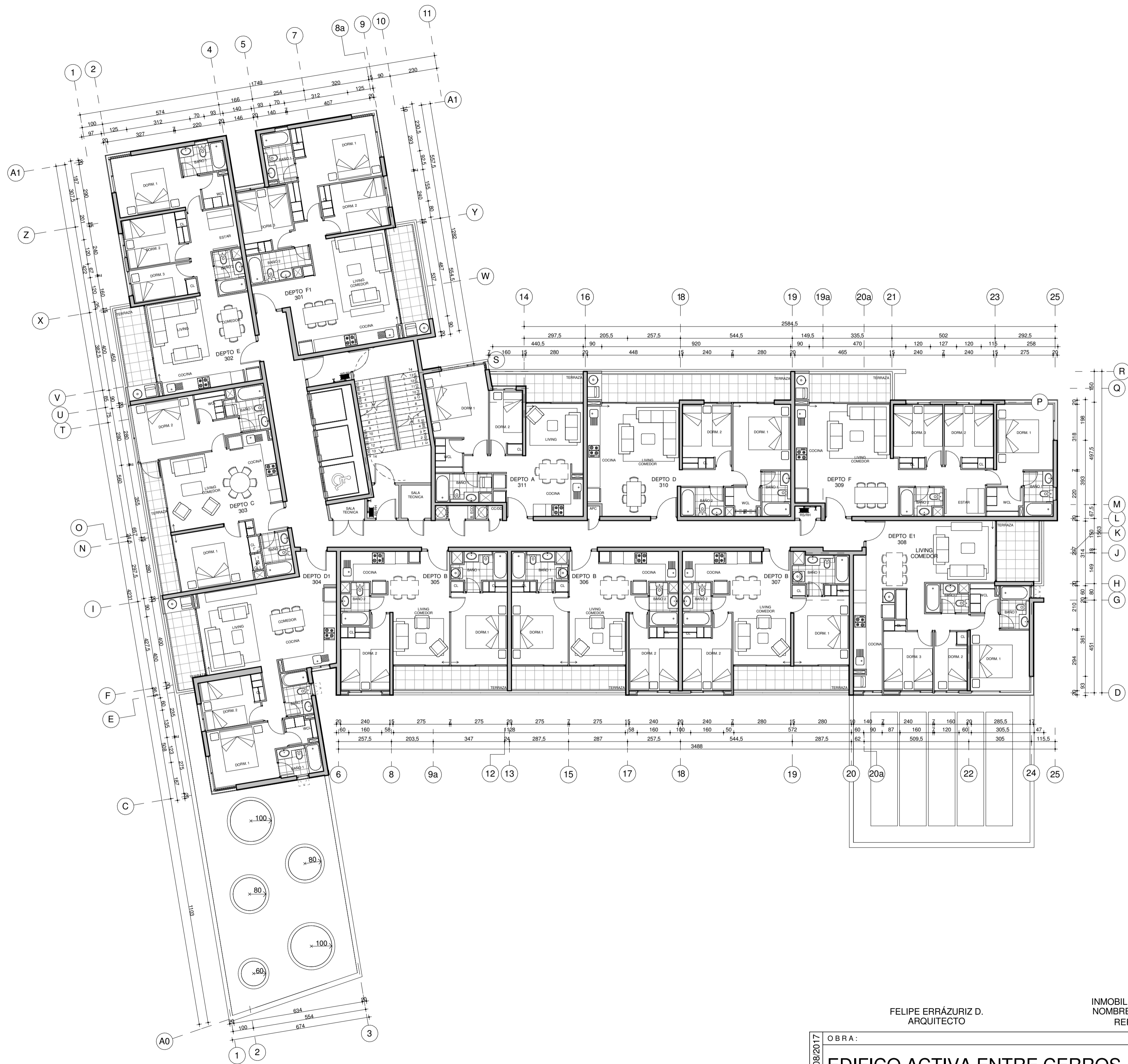
Planta General Piso 3
