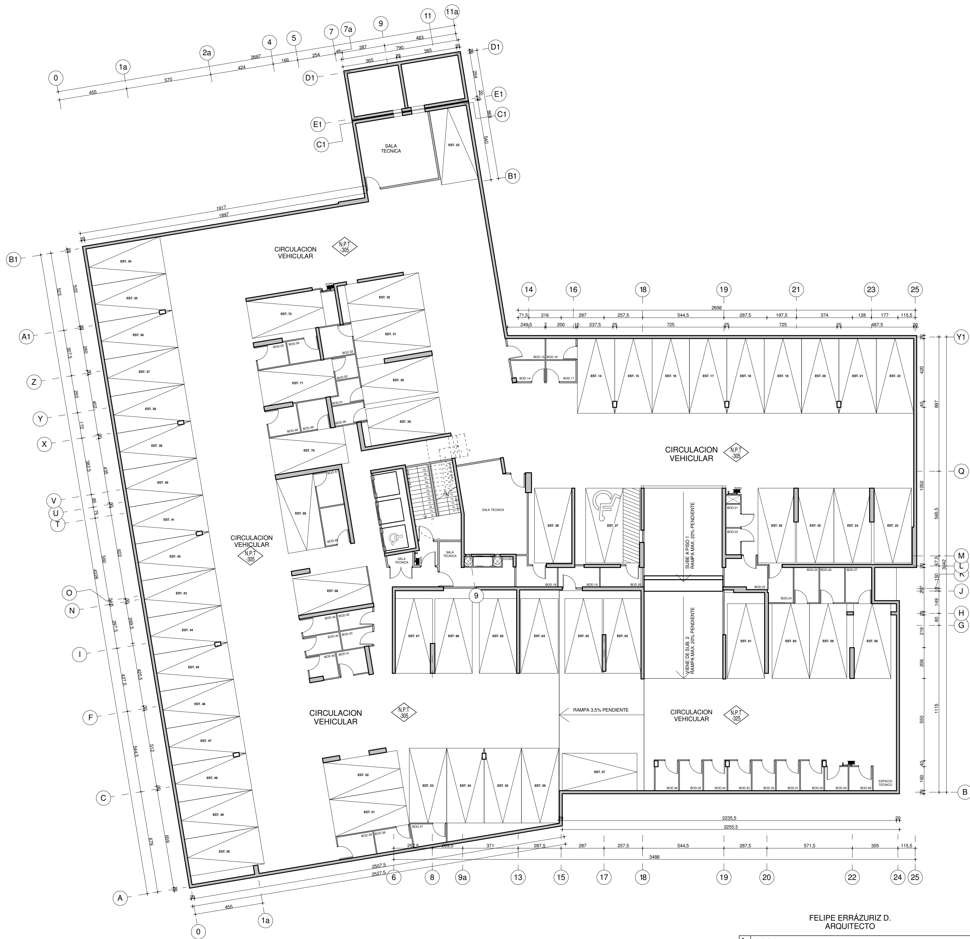
Planta General Sub.1
